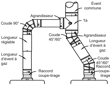
SCHÉMA 5 - Système d'évent combiné utilisant des pièces de type B en commençant par les raccords à coupe-tirage (C à B).
