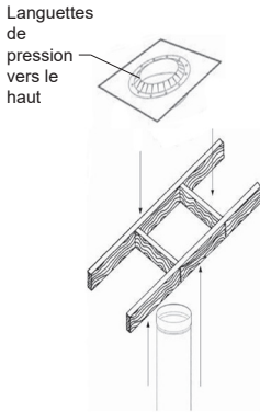
Schéma 13 - "Prise Rapide" - Coupe-feu/Plaque de support
